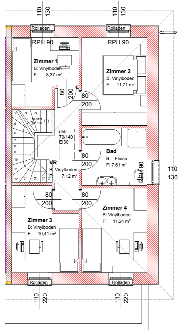
1. Obergeschoss 1:100
