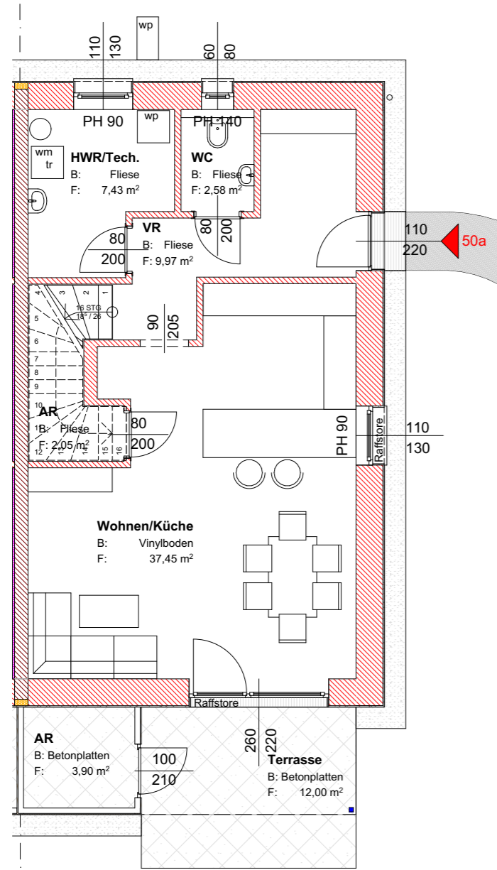
0. Erdgeschoss 1:100
