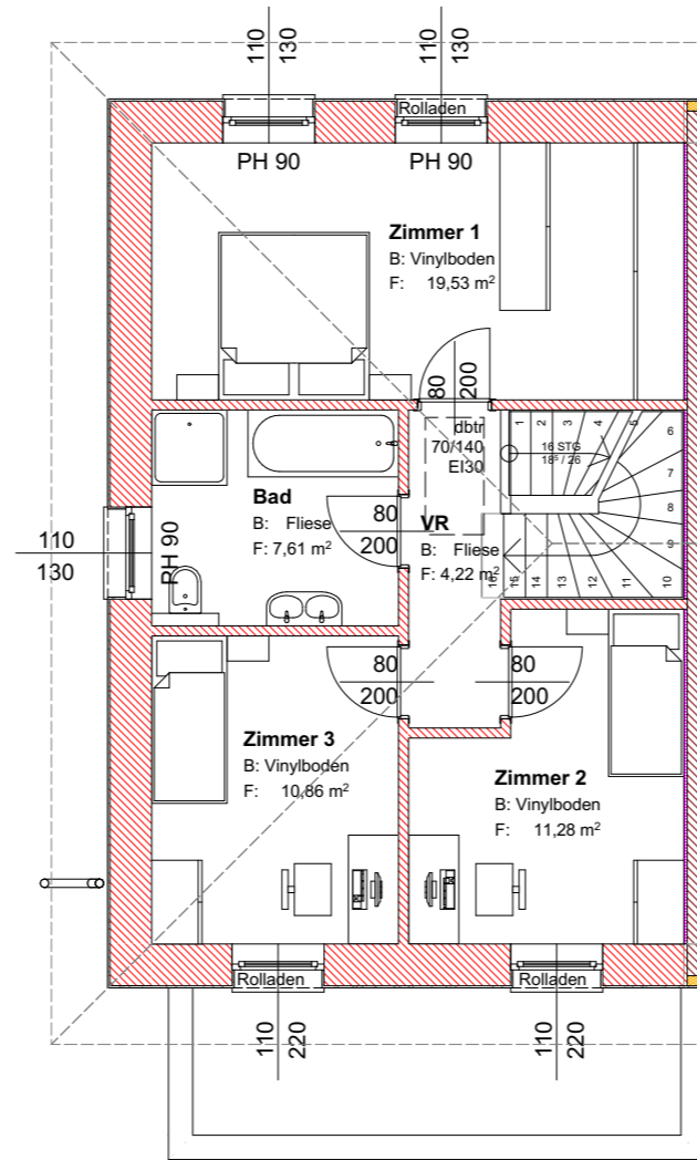
1. Obergeschoss 1:100
